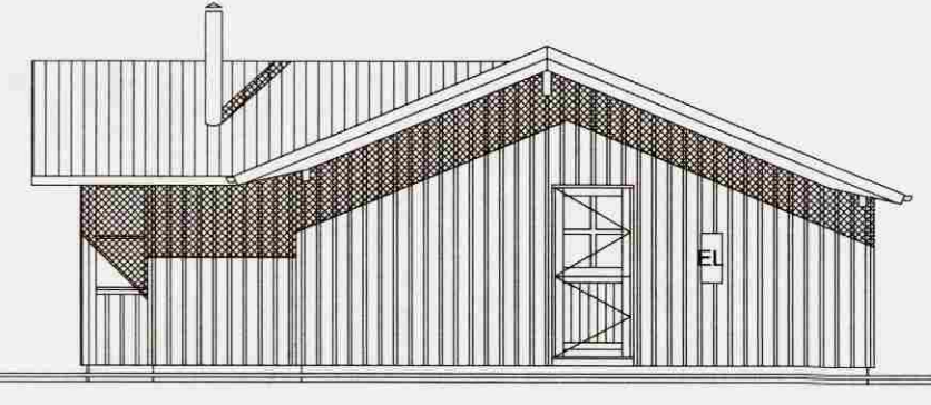
SUBAUSTUR 1:100
