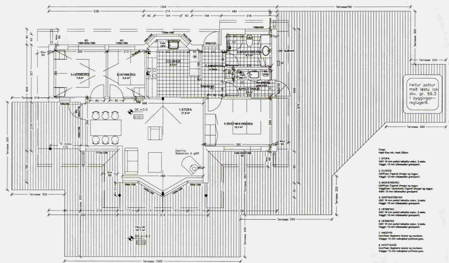
GRUNNMYND 1:100
