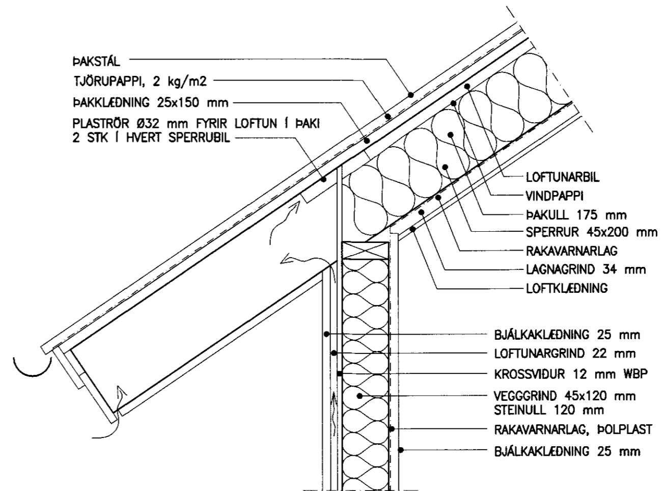
FRÁANGUR VID ÚTVEGG OG ÞAK 1:10
