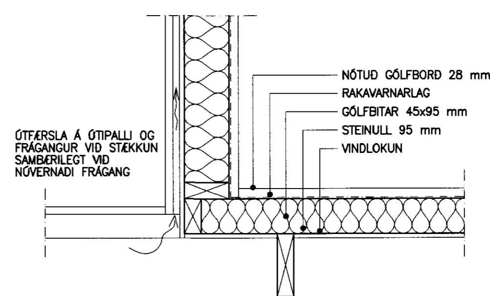
FRÁANGUR VID ÚTVEGG OG GÓLF 1:10
