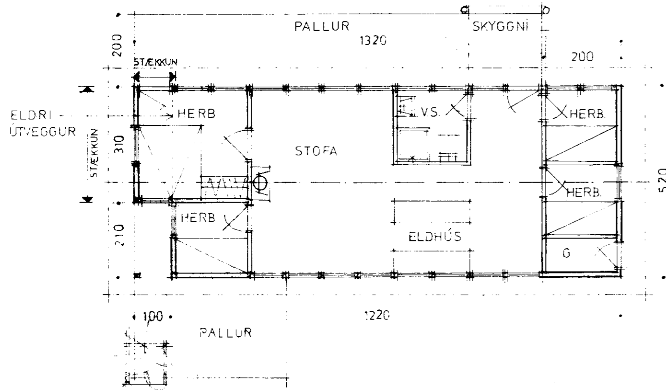
GRUNNMYND
