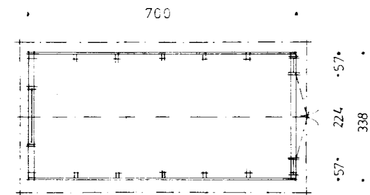
GRUNNMYND
