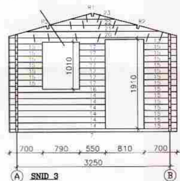
Skásagaðir bjálkar í göflum skrufast saman m. galv. tréskrúfum c/c 60 cm. sjá lið 18 á blaði nr. SN2
