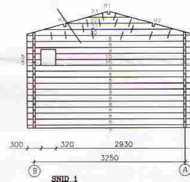
Skásagaðir bjálkar í göflum skrufast saman m. galv. tréskrúfum c/c 60 cm. sjá lið 18 á blaði nr. SN2
