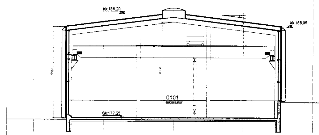
Sneiðing A-A
