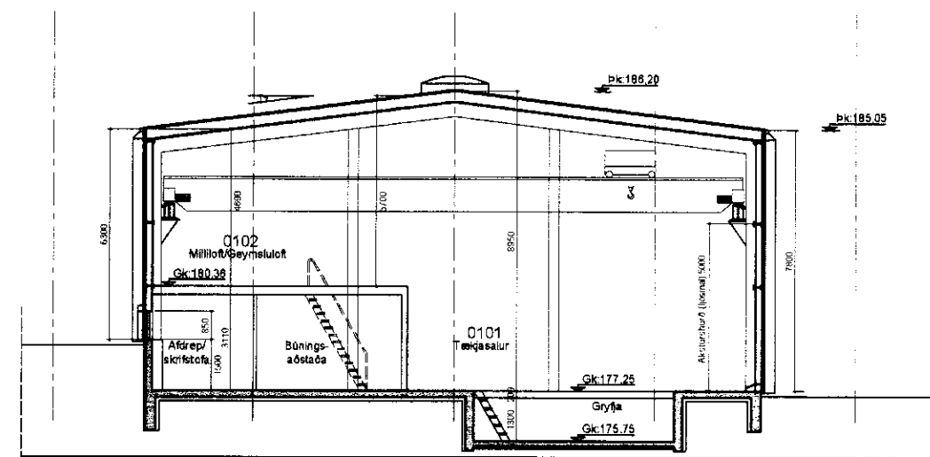
Sneiðing B-B
