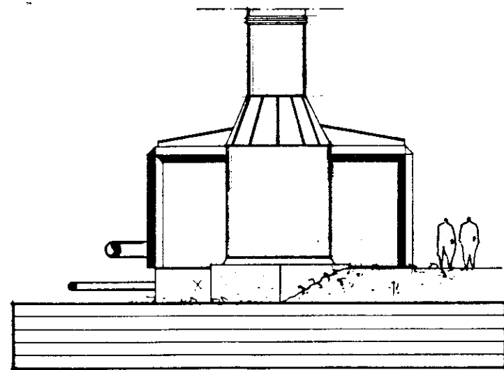
útlit nord-austur
