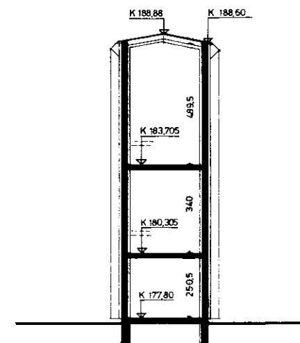
Sneiding G-G
