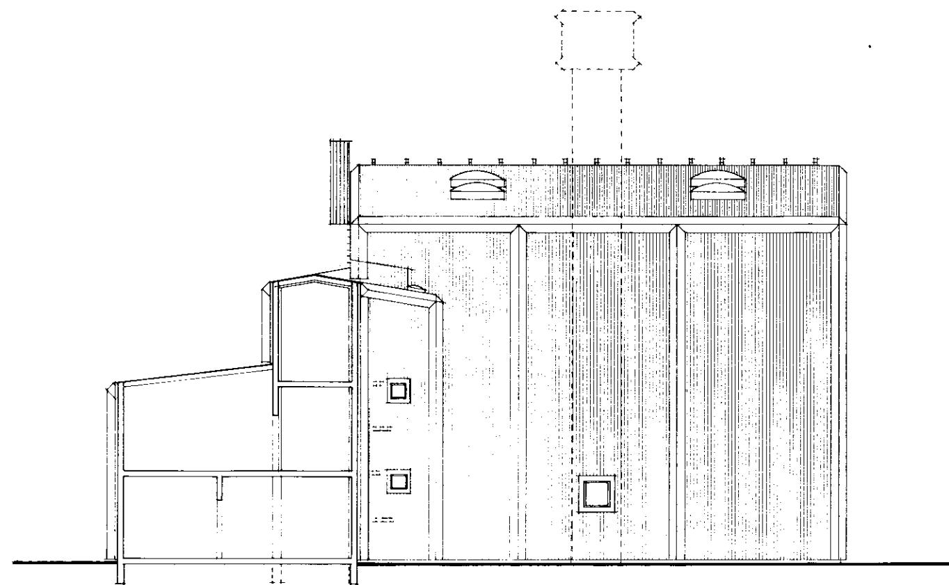
Sneiding F-F
