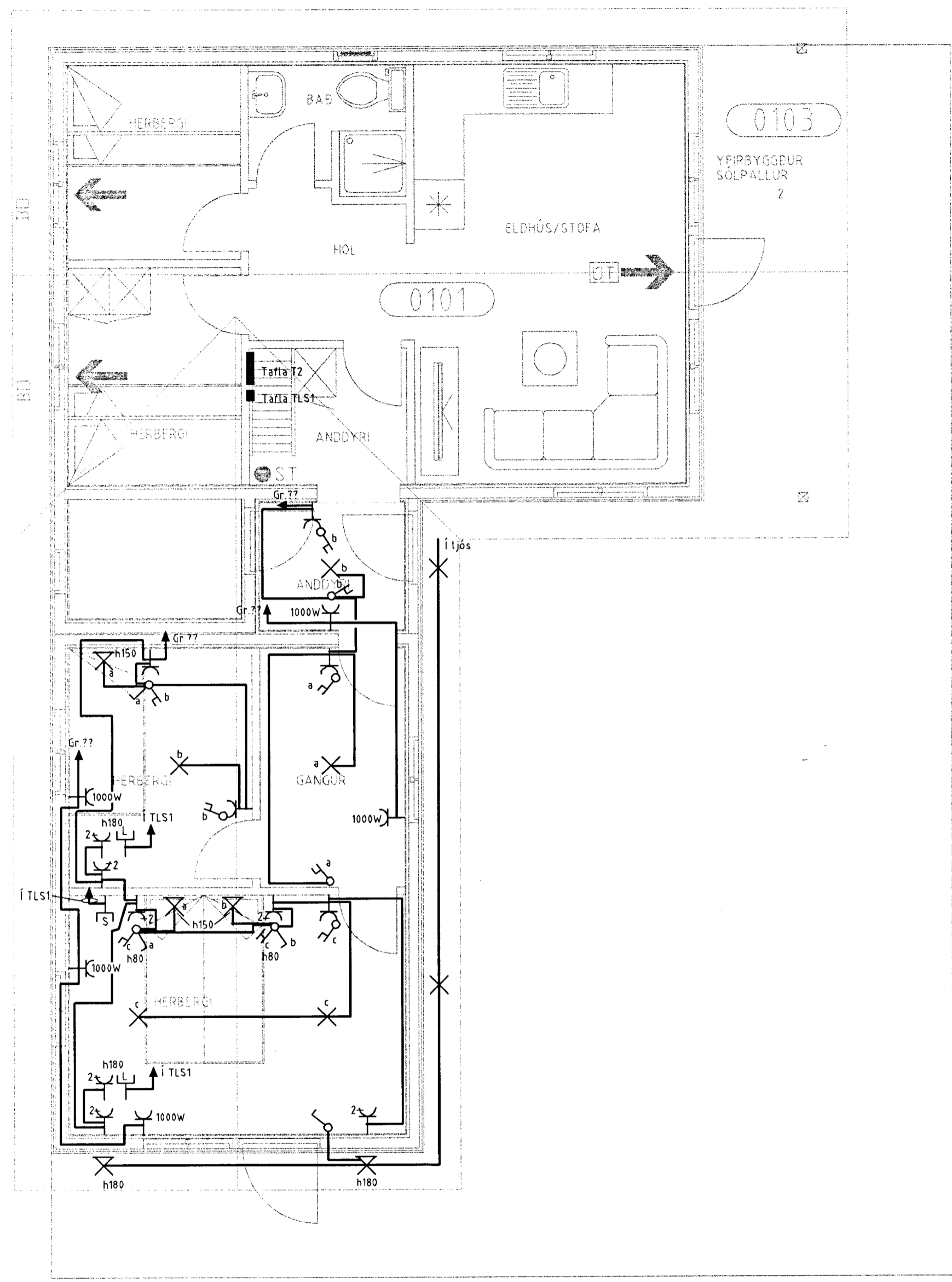
Grunnmynd raflagna
