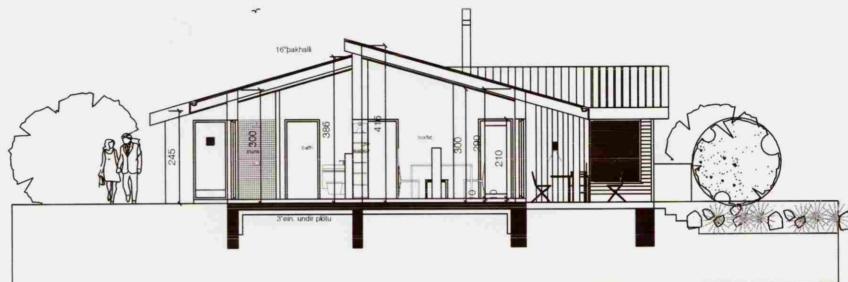
sneiðing A-A
