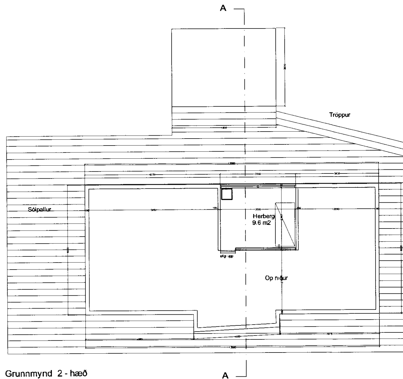
Grunnmynd 2 - hæð
