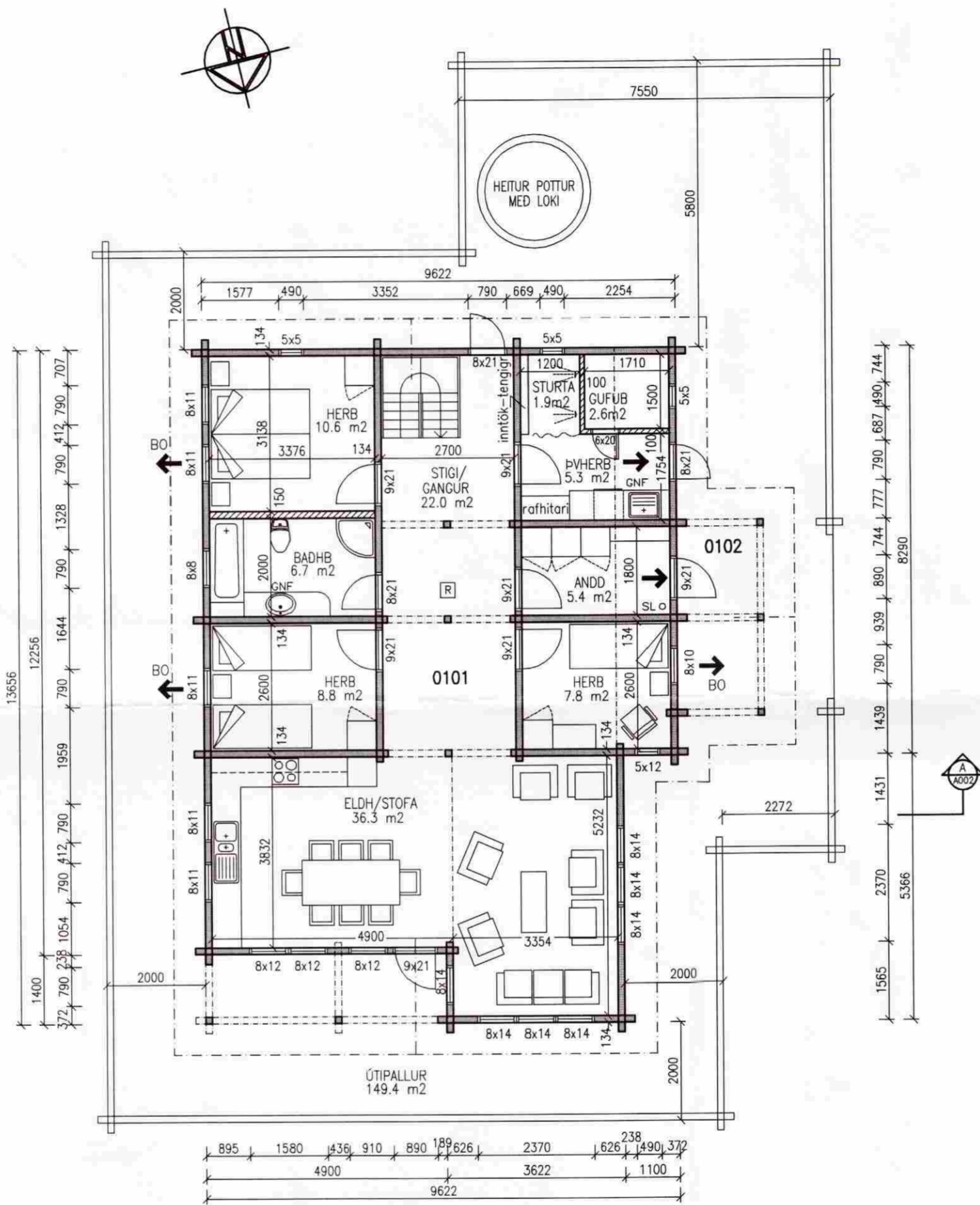
GRUNNMYND NEDRI HÆÐ 1:100
