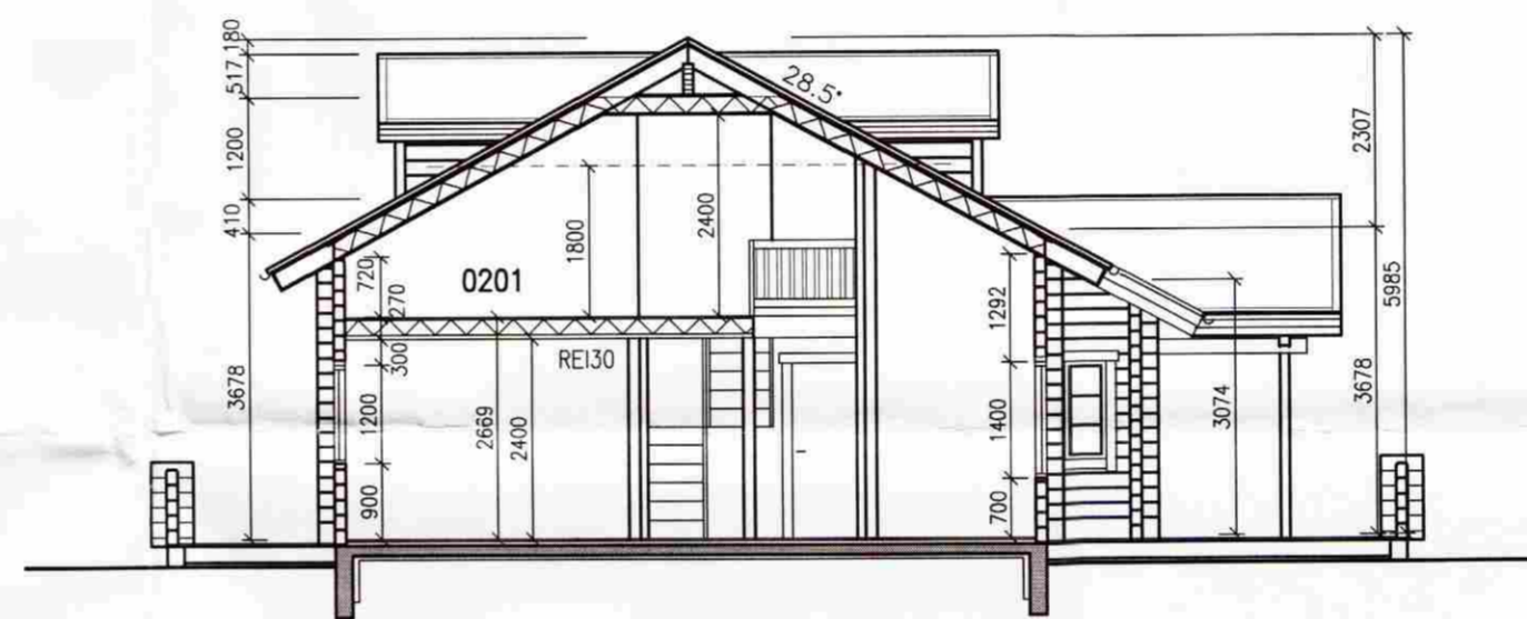
SNID A-A 1:100
