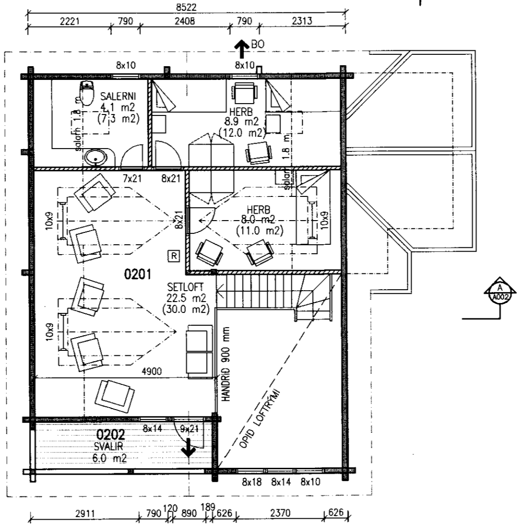
GRUNNMYND EFRI HÆÐ 1:100
