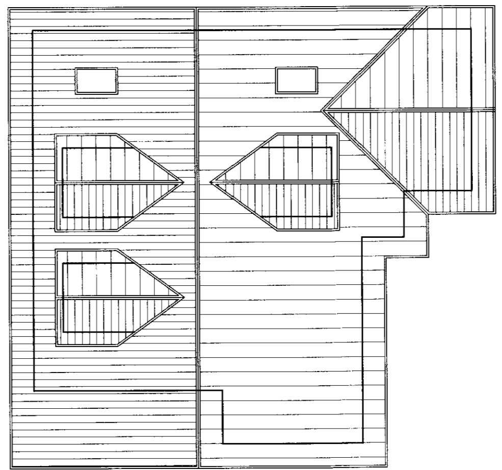
GRUNNMYND ÞAK 1:100
