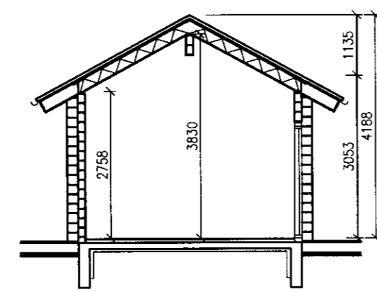
SNID B-B 1:100
