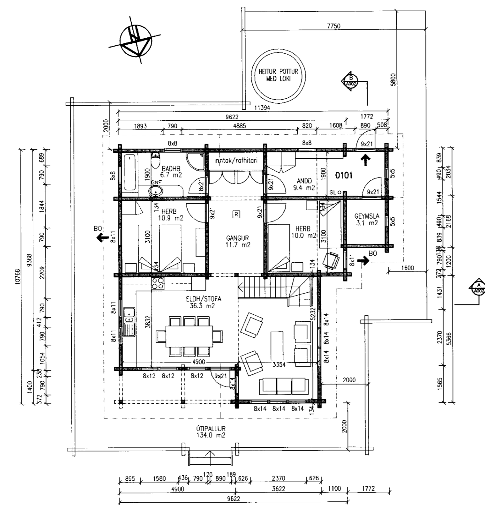
GRUNNMYND NEDRI HÆÐ 1:100
