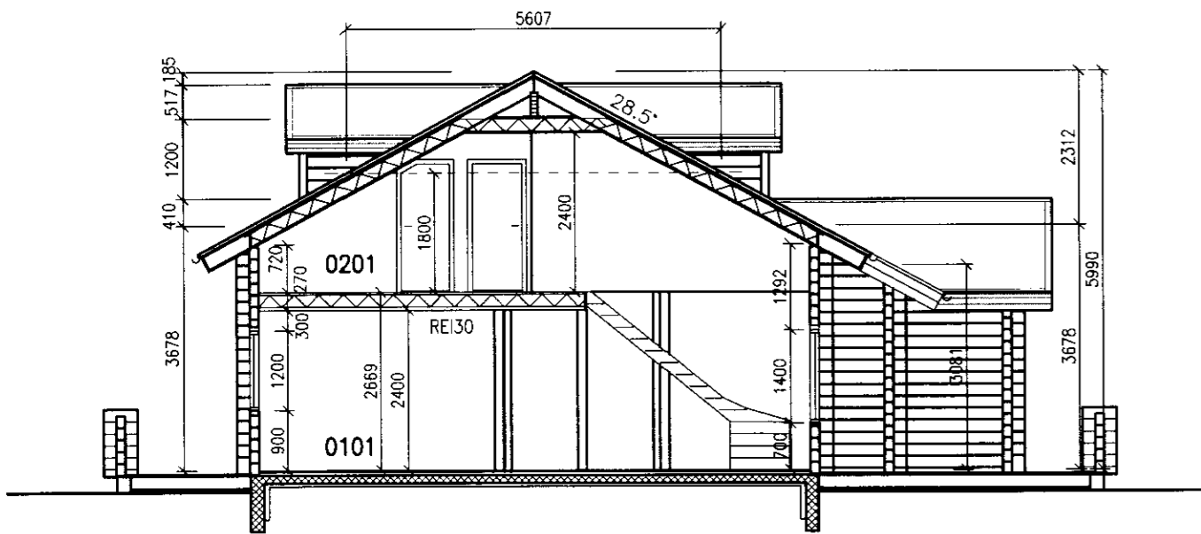
SNID A-A 1:100
