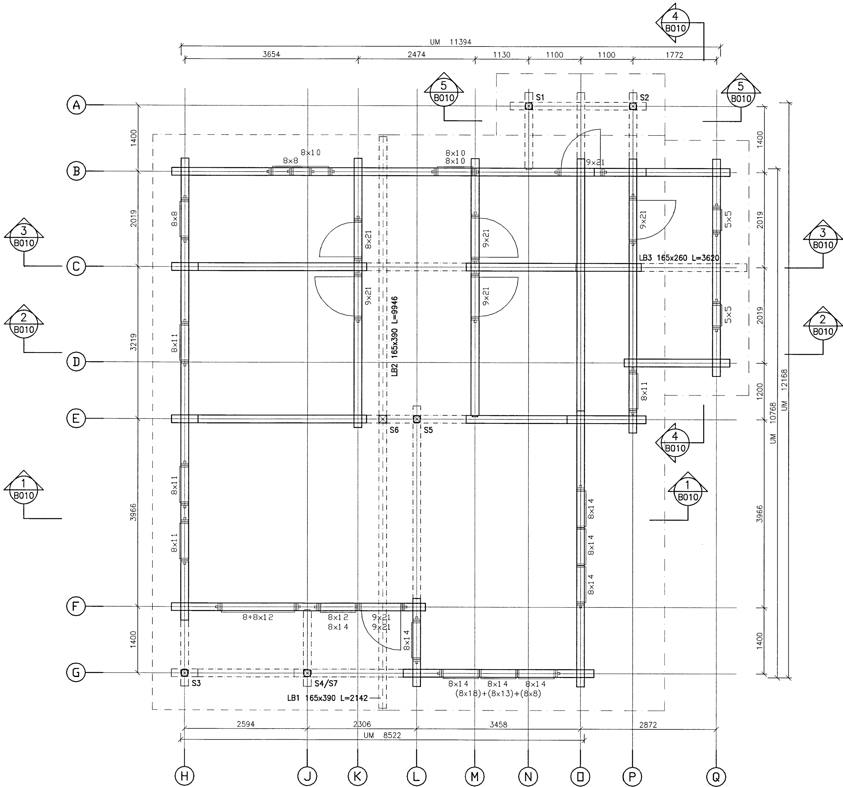
BJÁLKAVEGGIR GRUNNMYND 1:50
