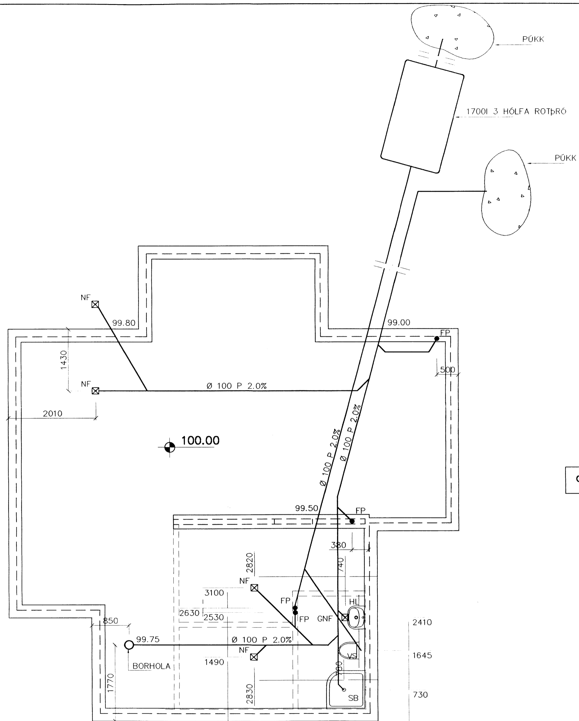
GRUNNMYND 1: 50
