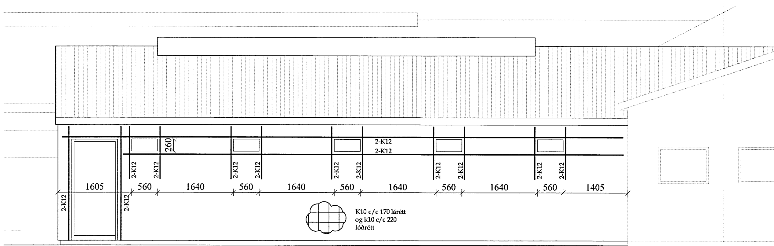
Útlit veggjabendingar í vestur mk. 1:50
