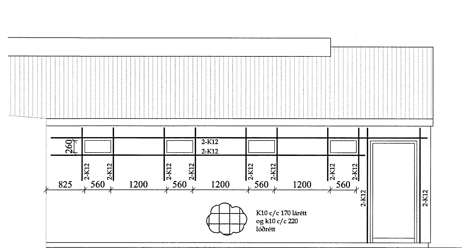
Útlit veggjabendingar í austur mk. 1:50
