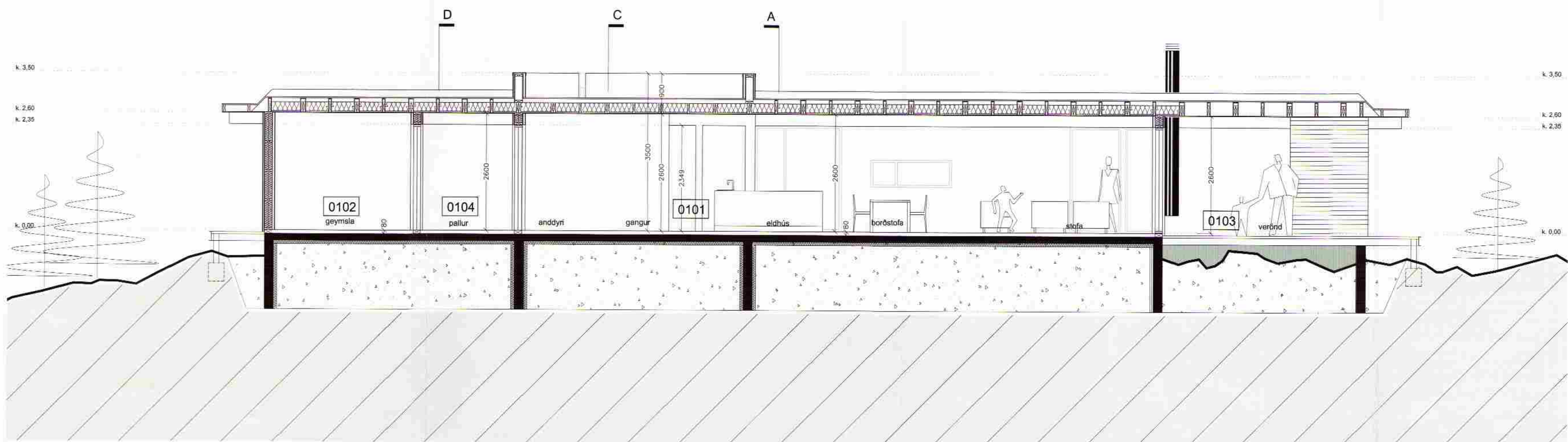
SNEIDING B - B M 1:50
