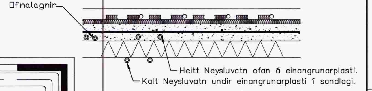
FRÁGANGUR LAGNA Í PLÖTU Í ÍBÚÐ MKV. 1:10
