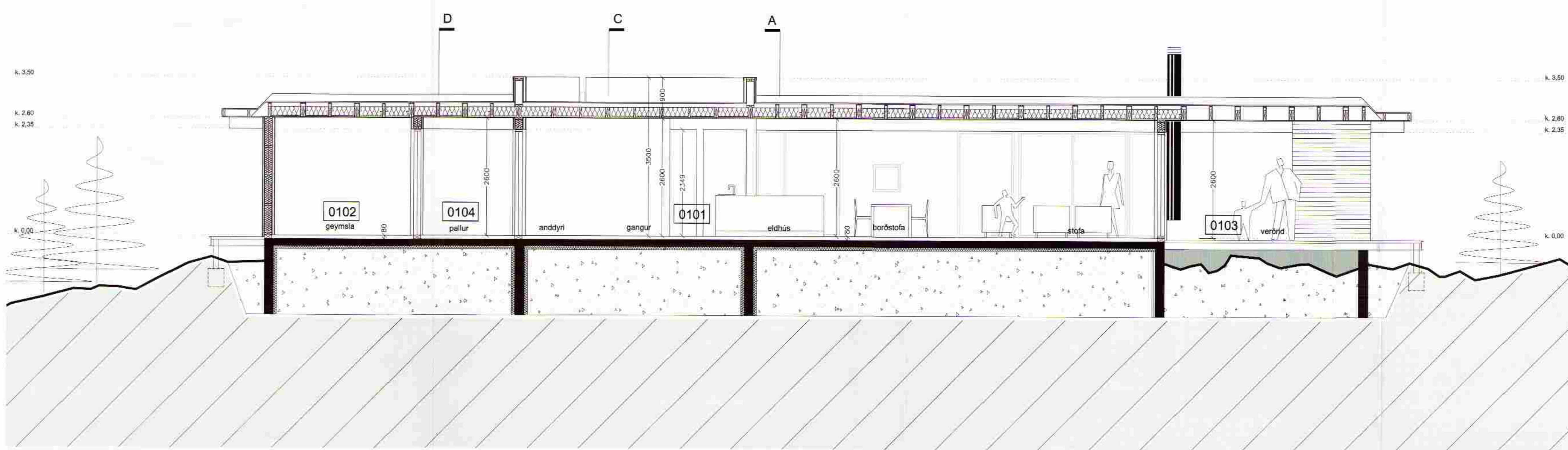
SNEIÐING B - B M 1:50
