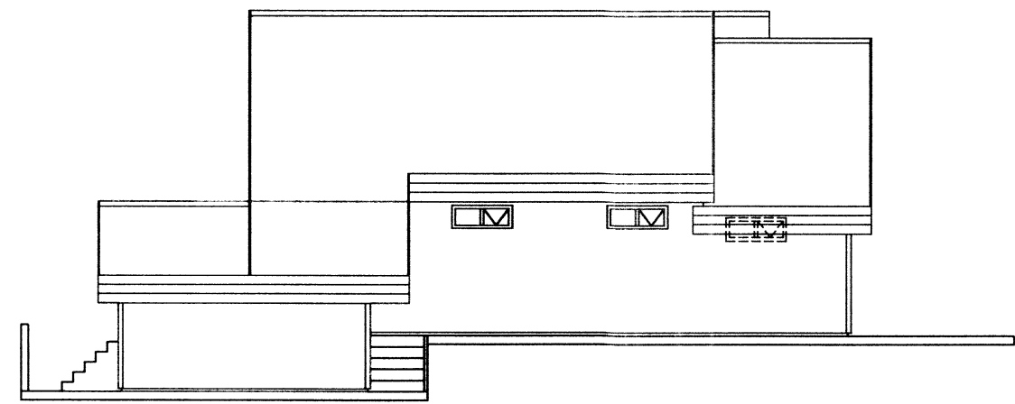
ÚTLIT SÚÐUR 1:100
