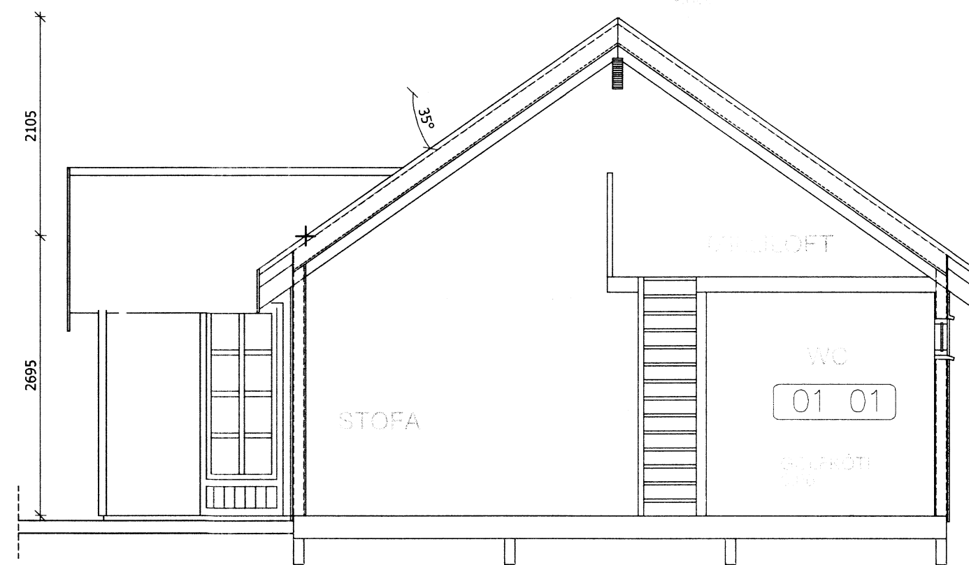
SNID A-A 1:50
