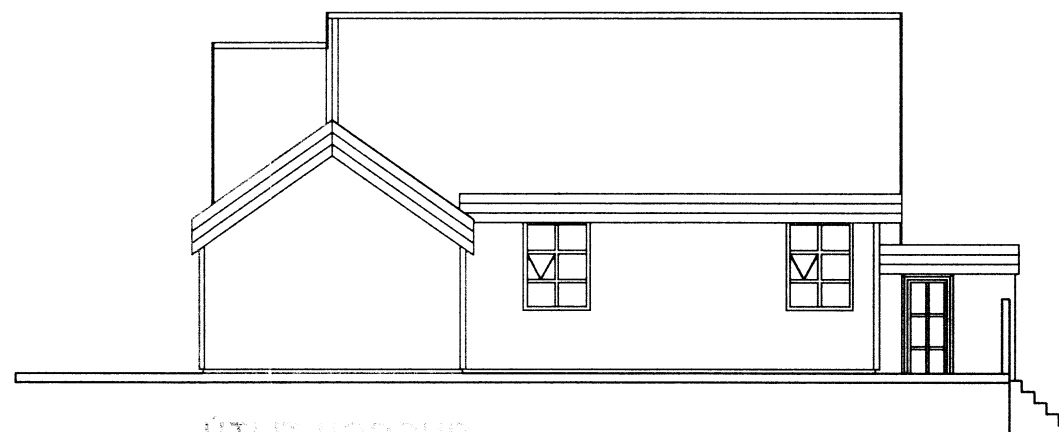
ÚTLIT NORÐUR 1:100
