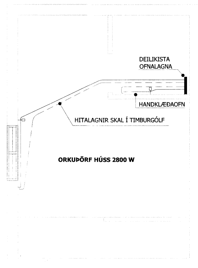
30 GRUNNMYND OFNALAGNA Mkv 1:50
