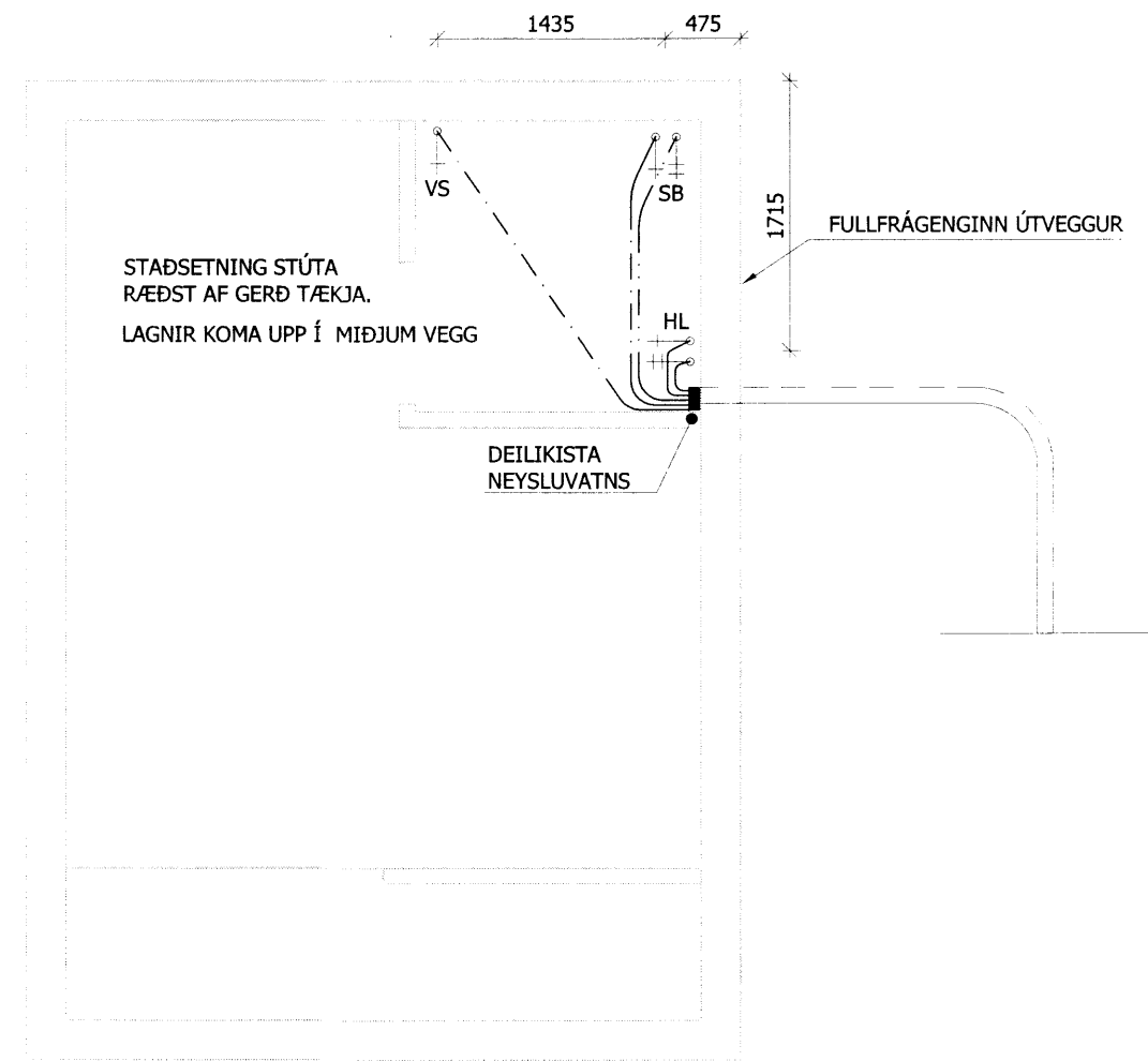
32 GRUNNMYND NEYSLUVATNSLAGNA Mkv 1:50
