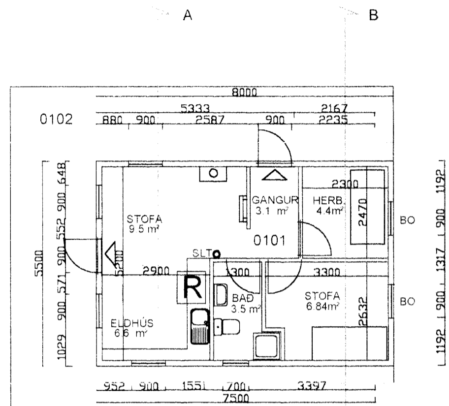
GRUNNMYND NEDRI HÆÐAR Mkv. 1 : 100
