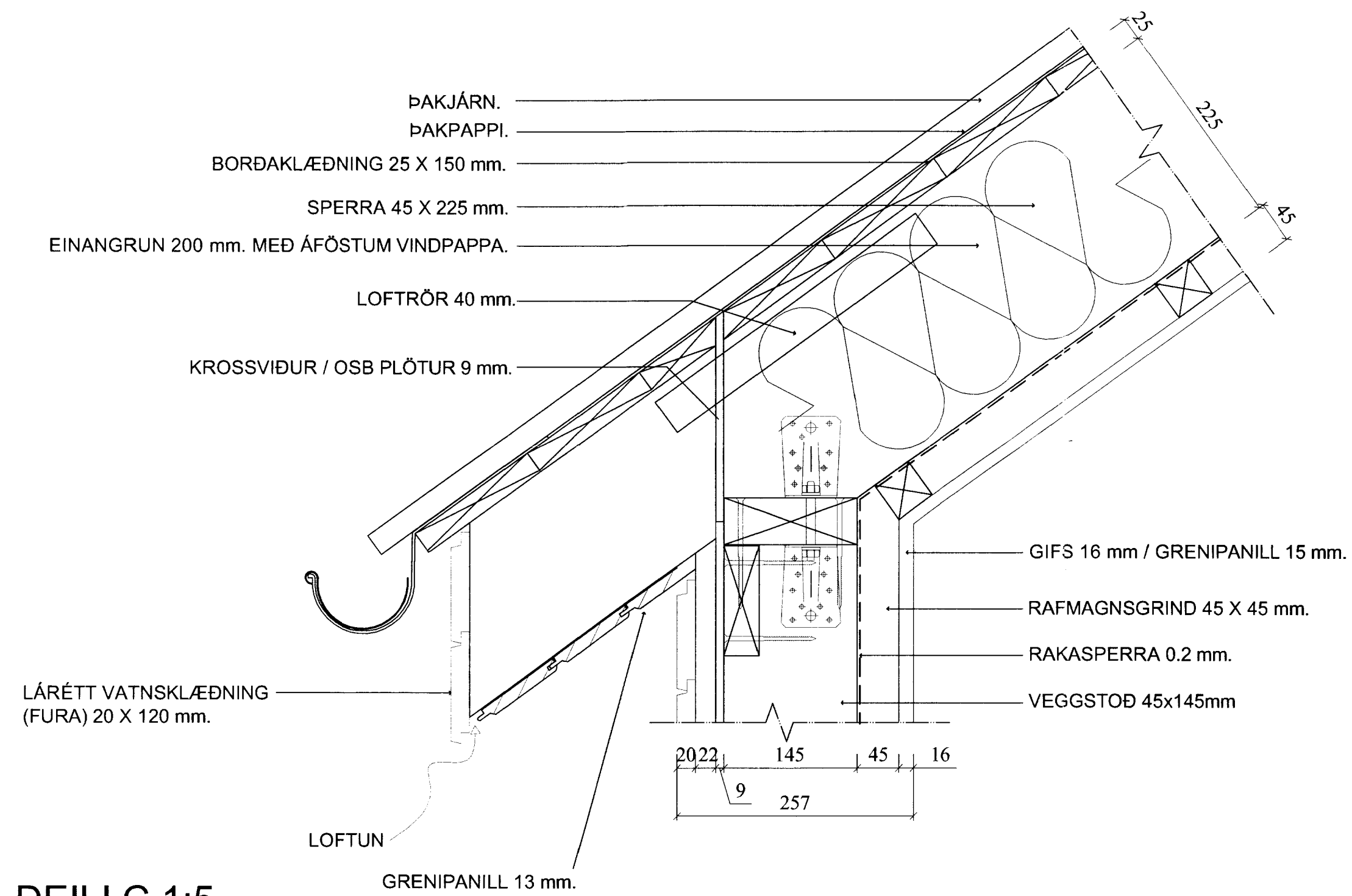
DEILI C 1:5 ÞAK, LÓÐRÉTT SNIÐ
