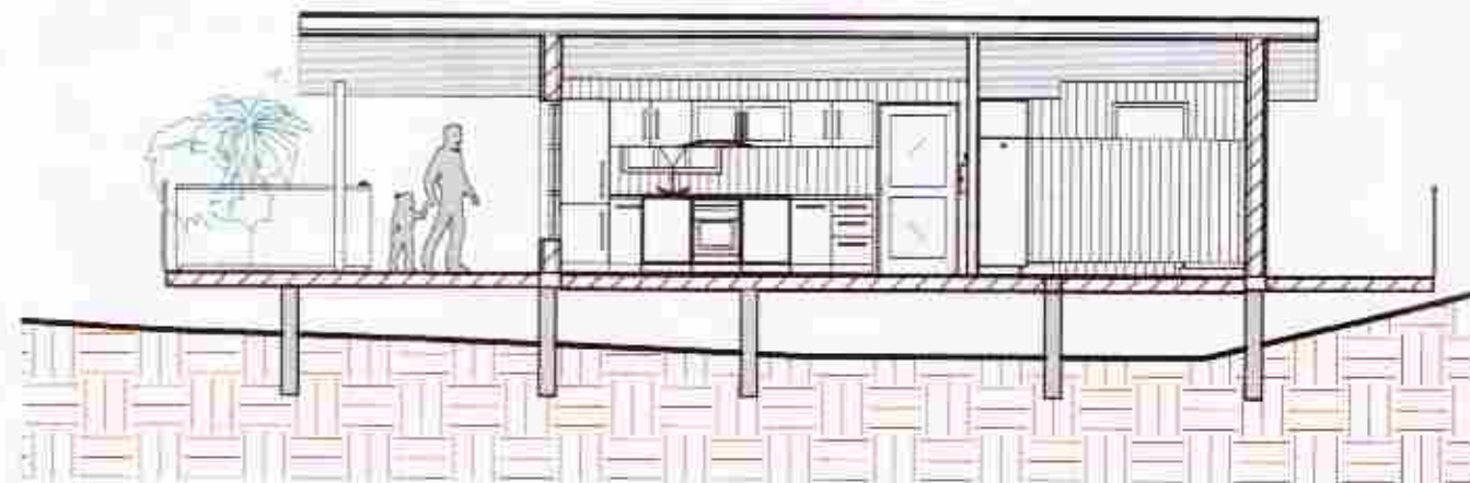
2 Snið 4 1 : 100
