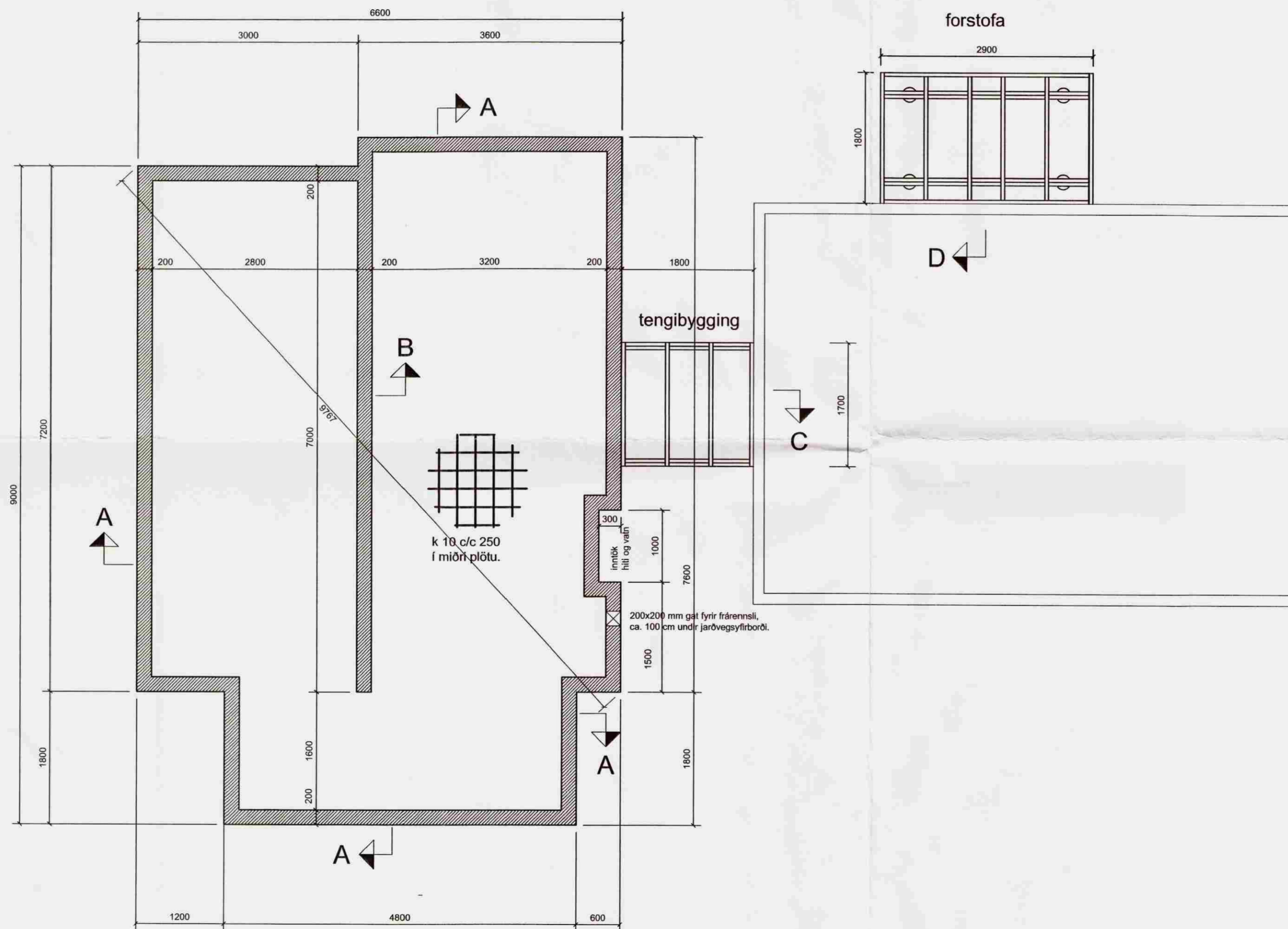
grunnmynd 1:50
