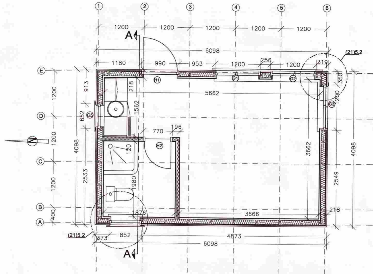
Grunnmynd
