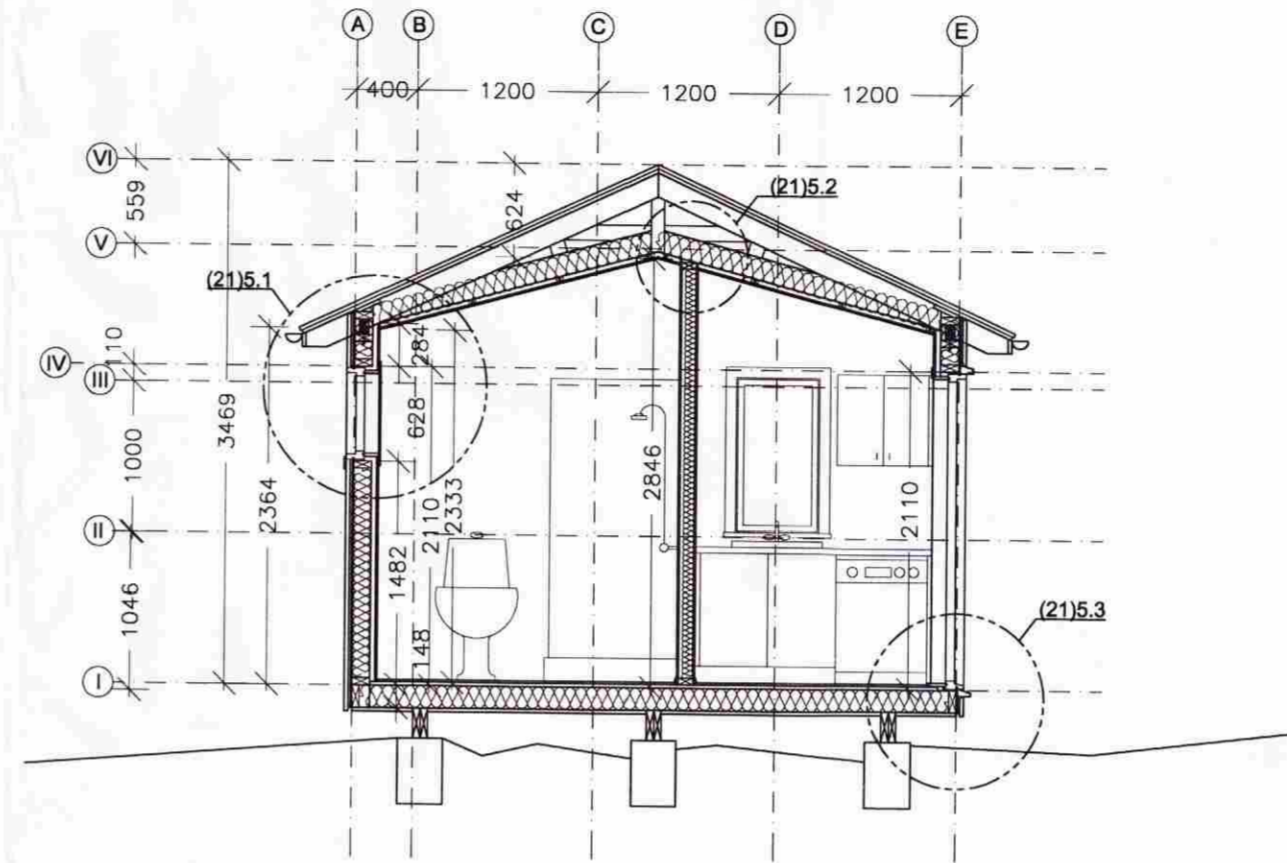
Snið A-A
