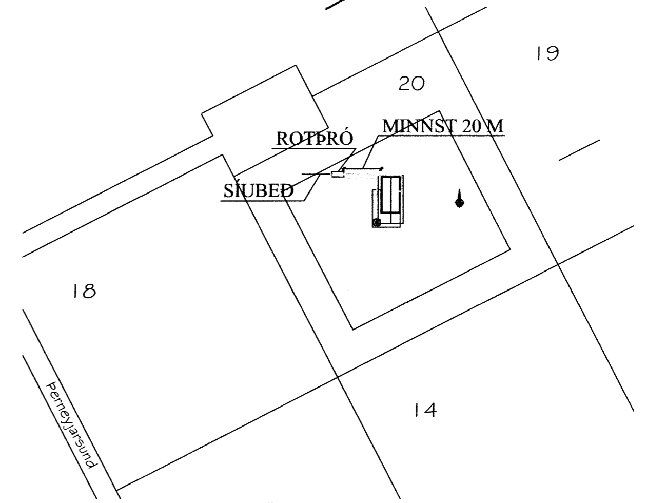
AFSTÖÐUMYND 1:1000
