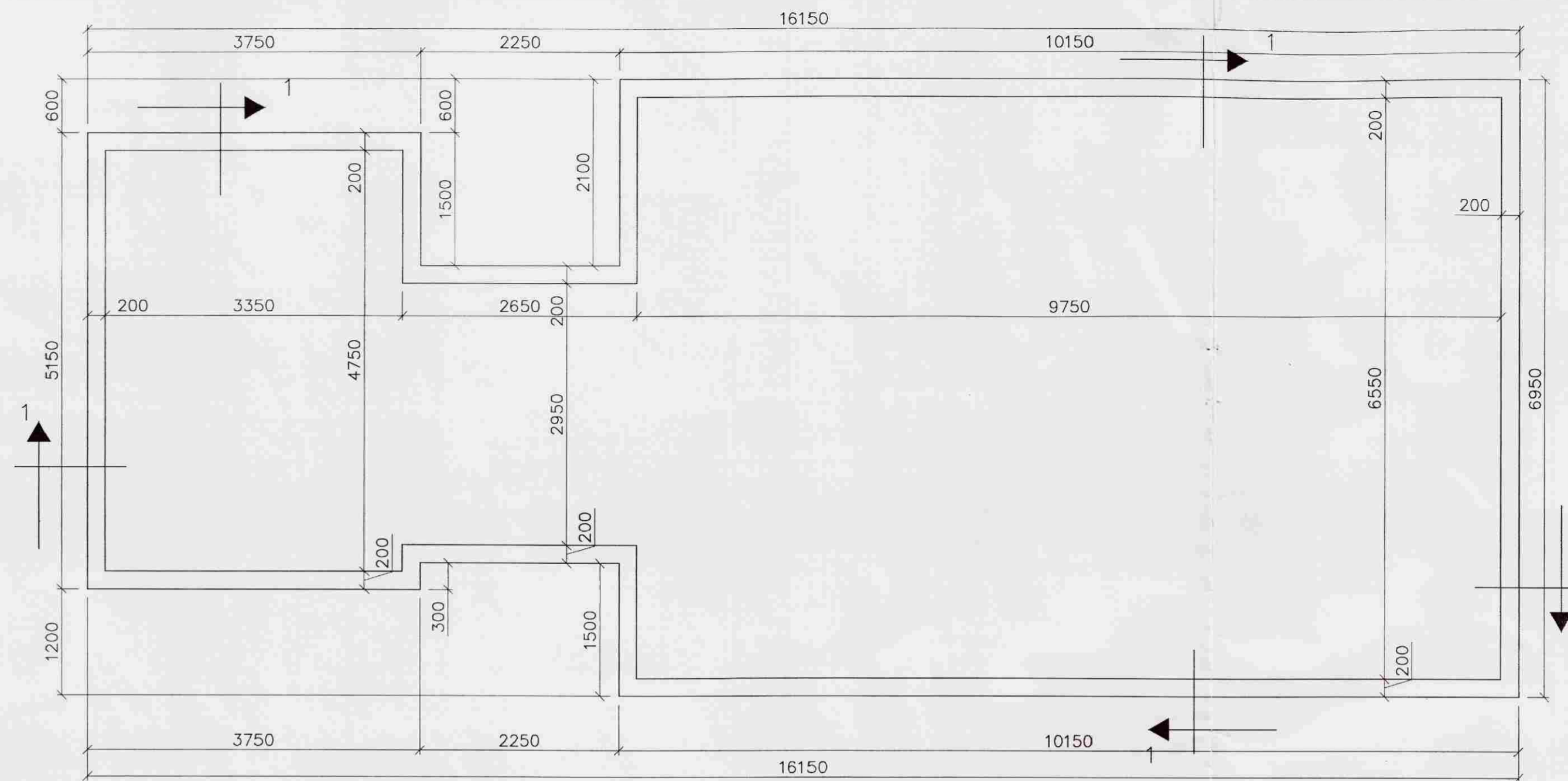
GRUNNMYND 1:50
