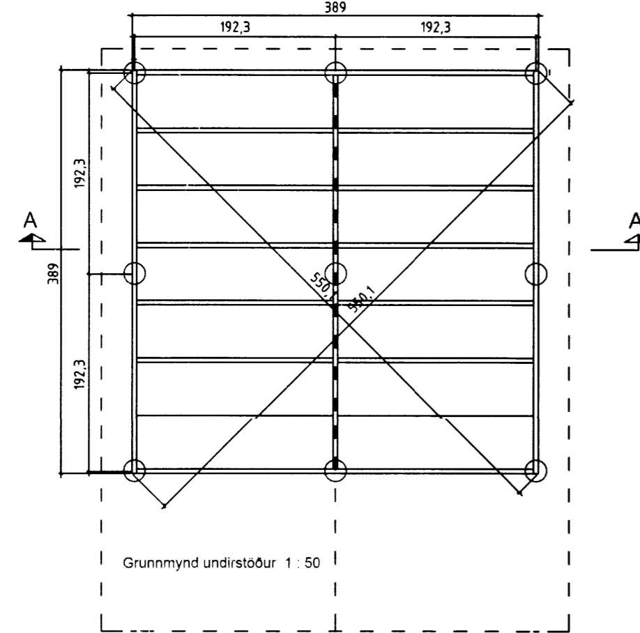
Grunnmynd 1 : 50
