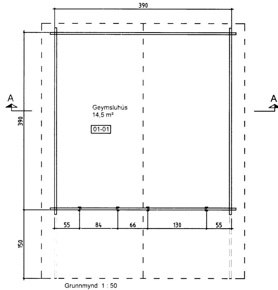
Grunnmynd 1 : 50
