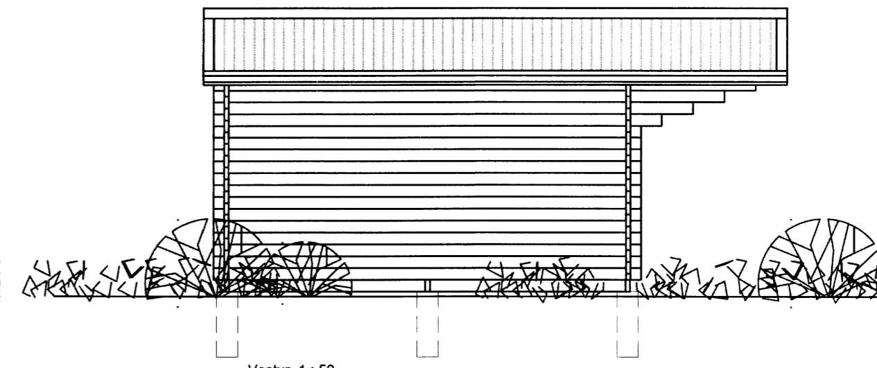
Vestur 1 : 50
