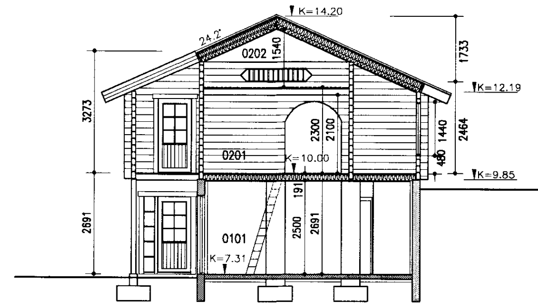
SNID A-A 1:100
