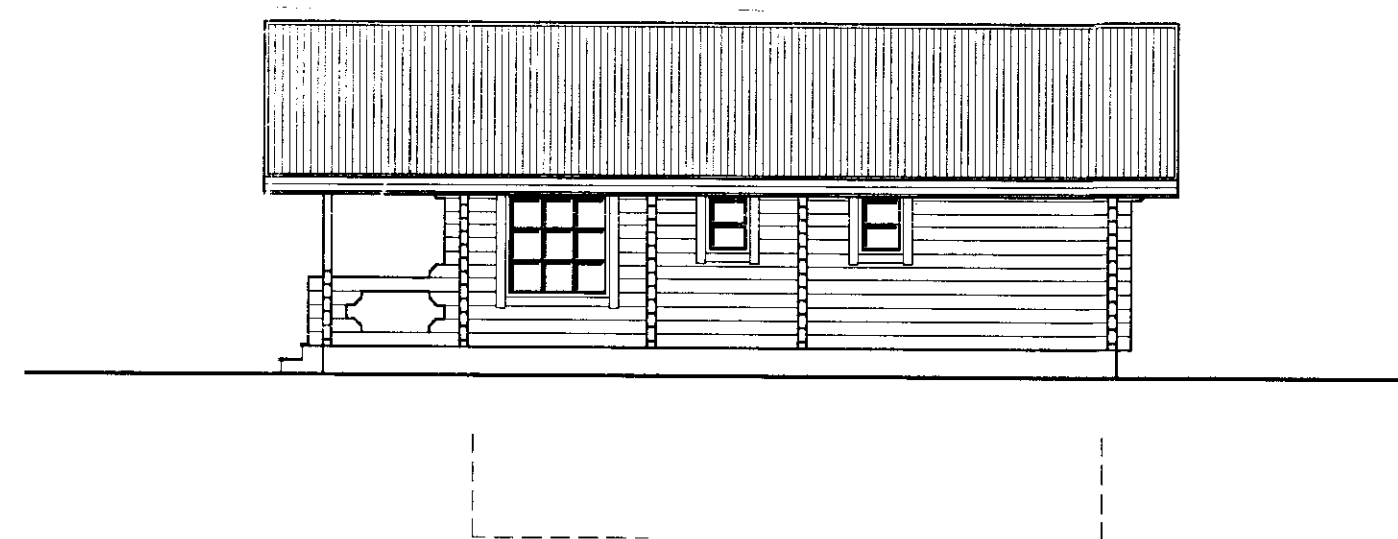
ÚTLIT NORDVESTURHLIÐ
