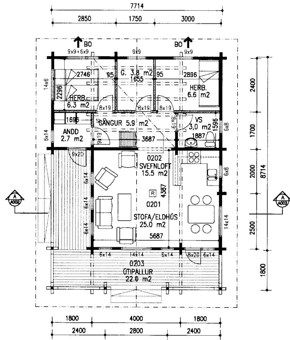
GRUNNMYND 2. HÆÐ
