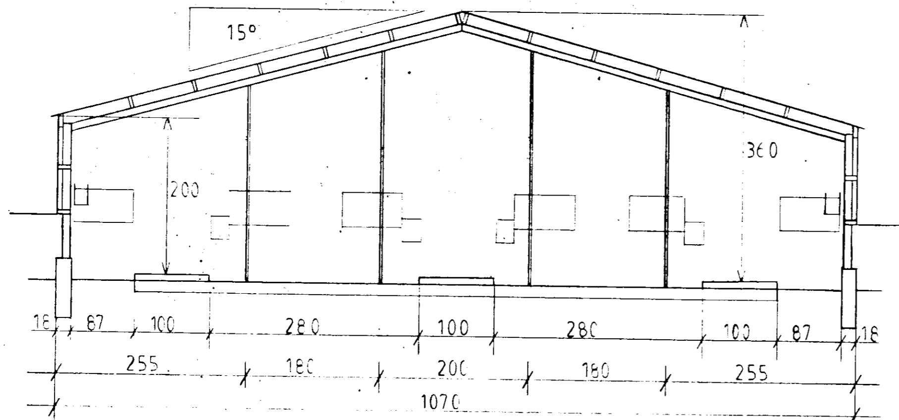
Snið A-A
