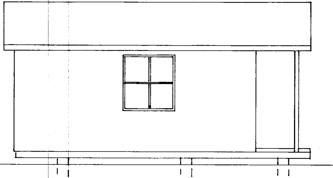
AUSTURHLIÐ
