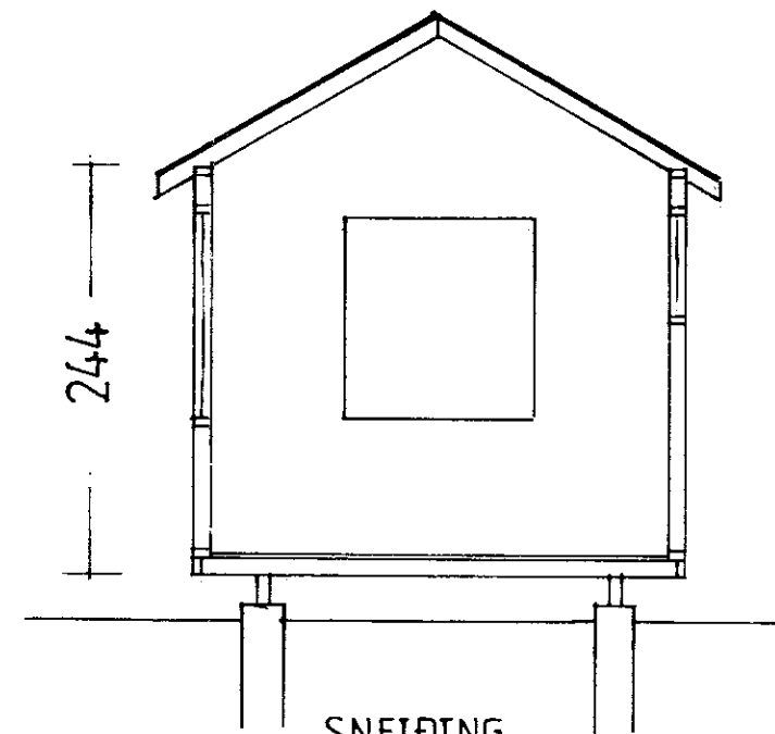
SNEIÐING
