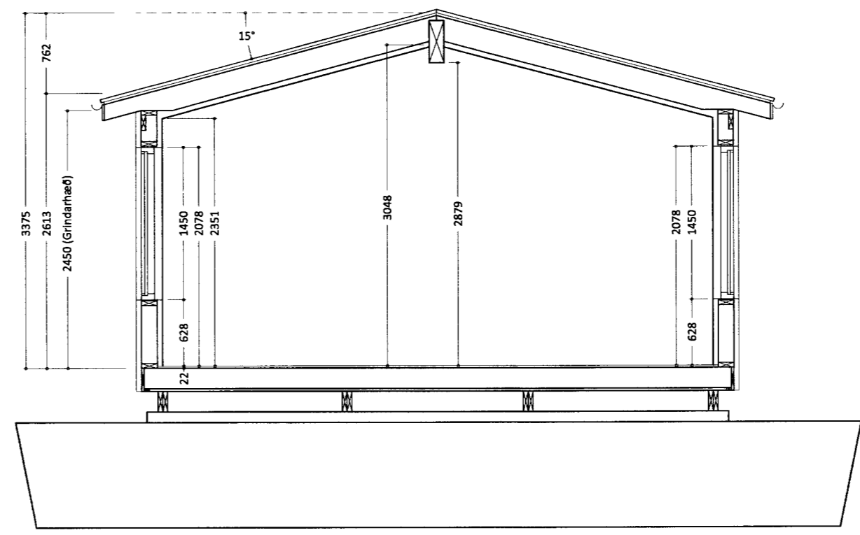
SNID A-A Mkv. 1:50
