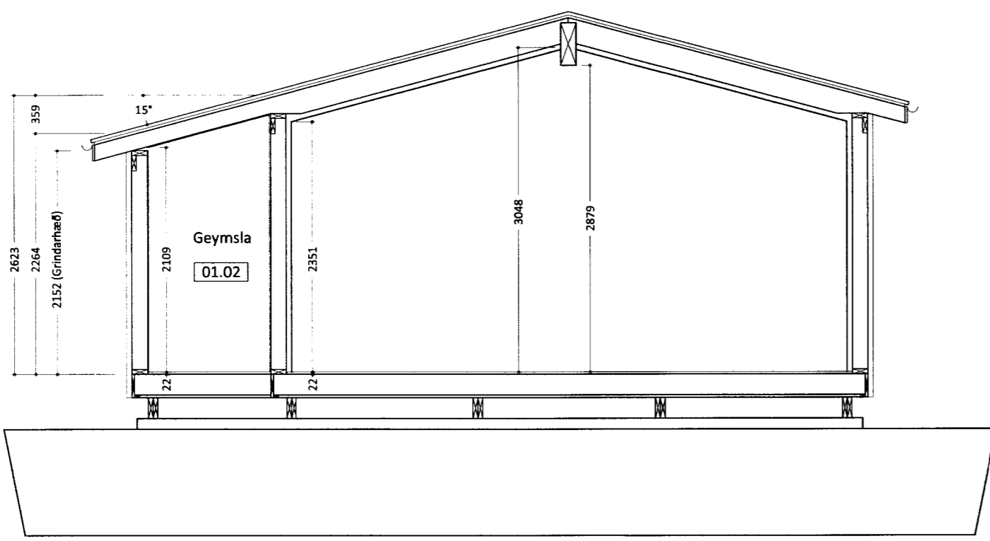
SNID B-B Mkv. 1:50
