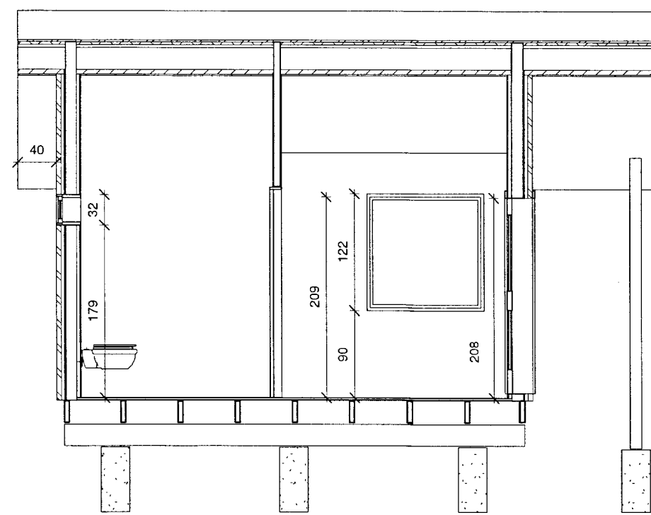
3 Snið-3 1 : 50
