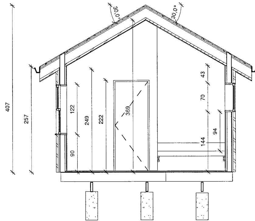
2 Snið-2 1 : 50
