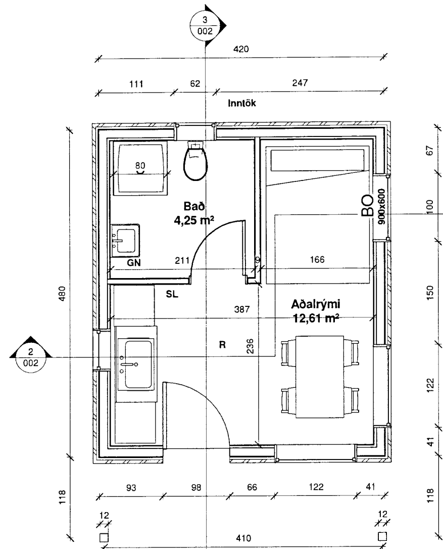
1 02-Hæð 1 1 : 50
