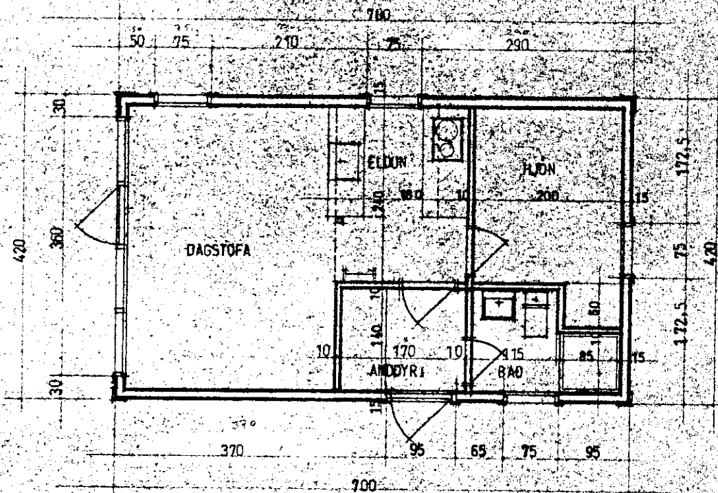
GRUNNMYND 1:50
