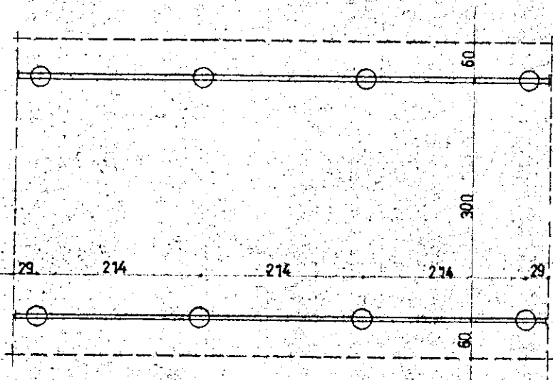
UNDIRSTOÐUR 1:50
