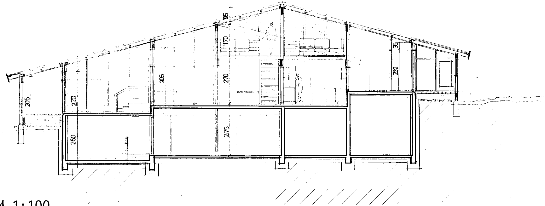
SNEIDING A-A M. 1:100
