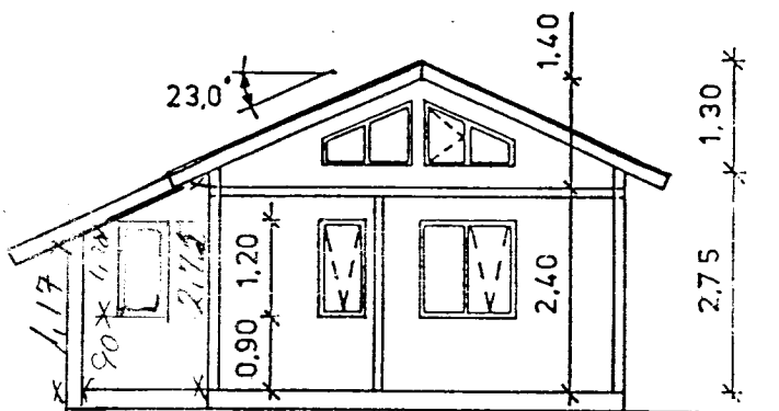
Snið A-A 1:100
