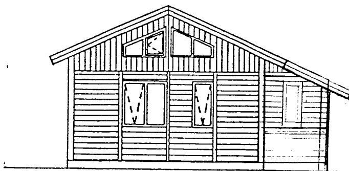
Norðlæg hlið 1:100
