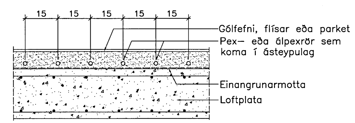
Snið í gólf 1:10
