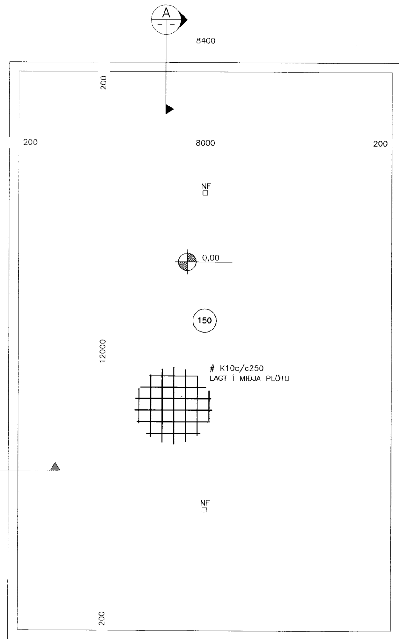
GRUNNMYND SÖKKULS 1:50
