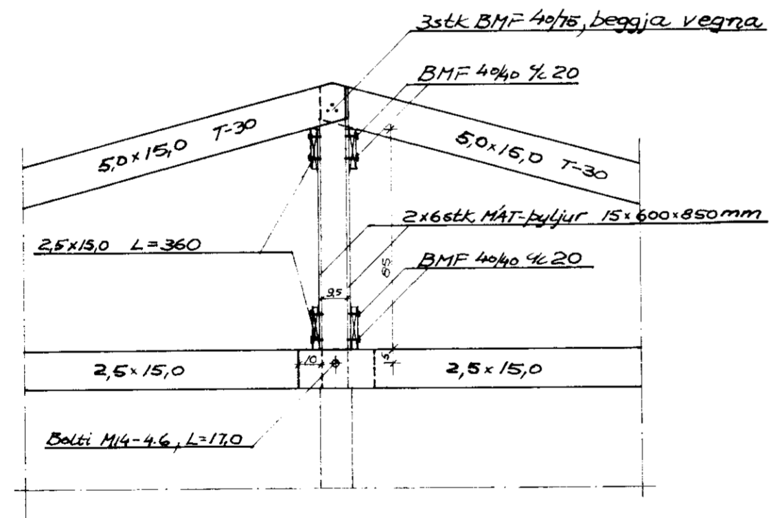
Snid B-B 1:20
