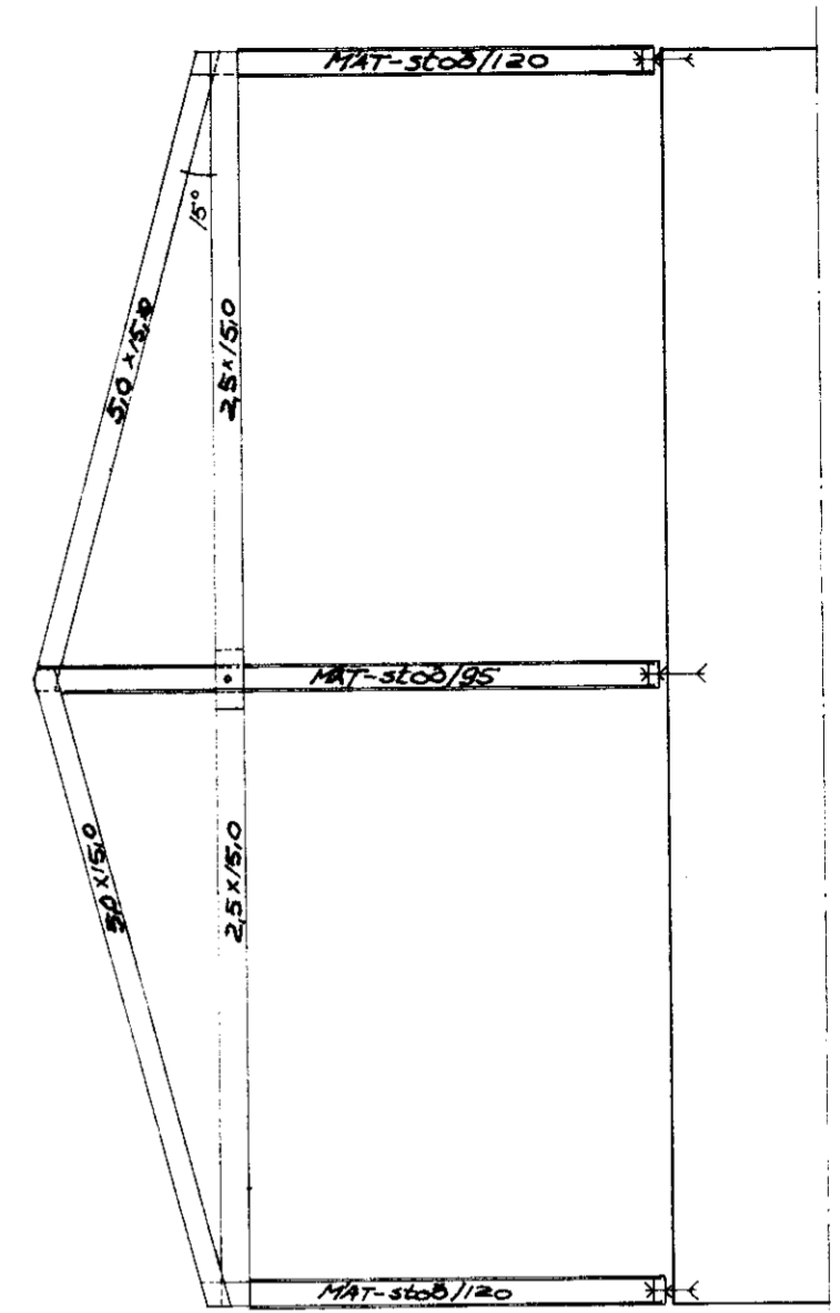
Snid A-A 1:50
