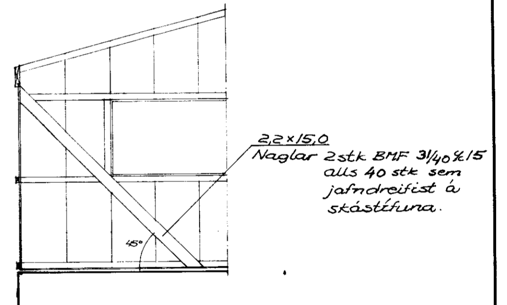
Stífung horna 1:50
