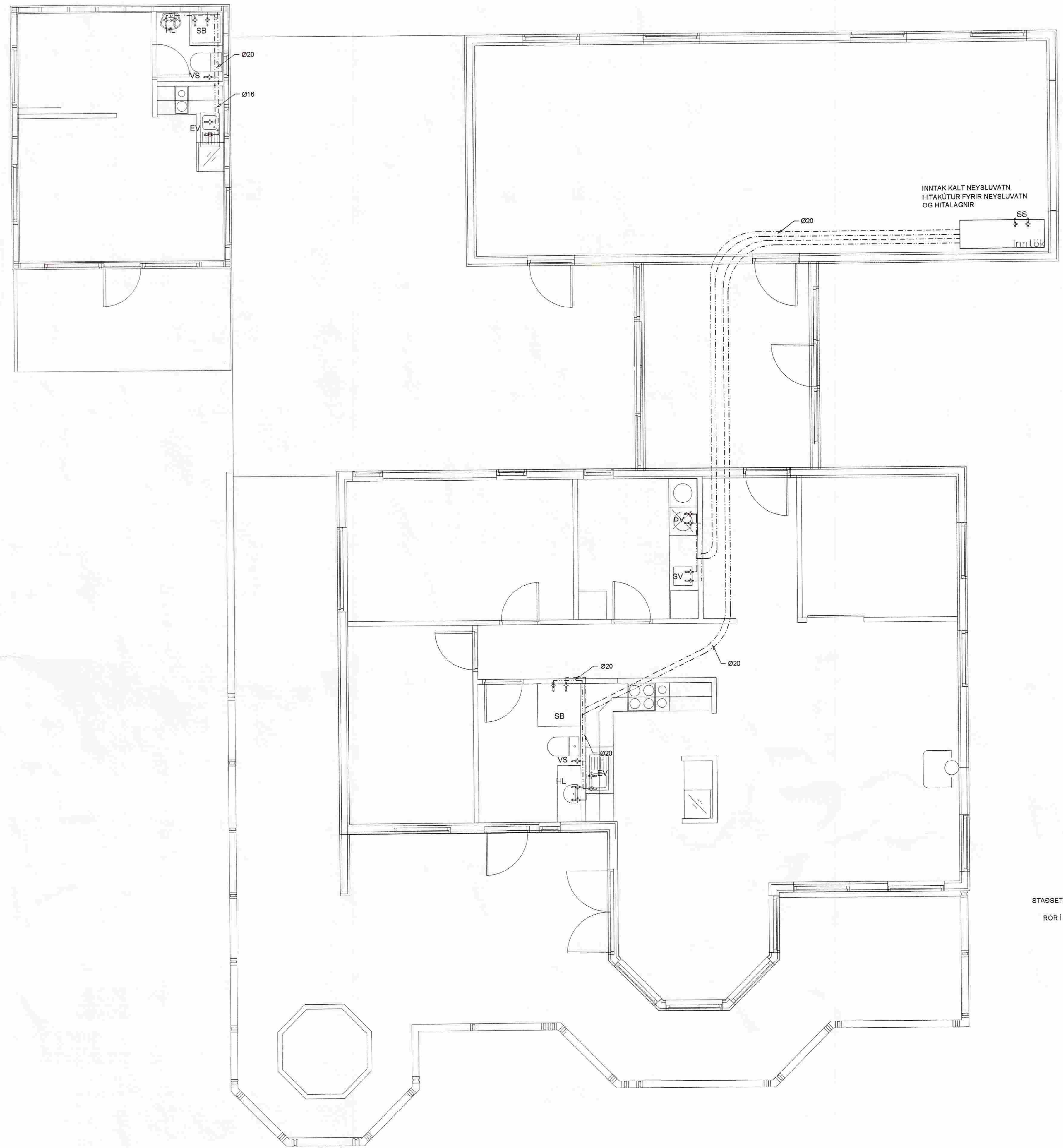
GRUNNMYND NEYSLUVATNSLAGNA, 1:50
