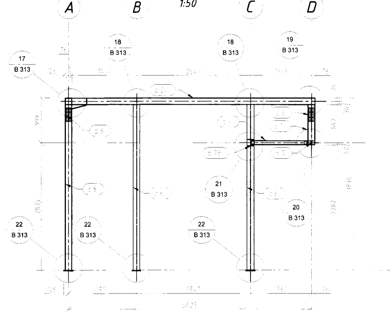
Mátlína 9 Ásýnd 1:50
