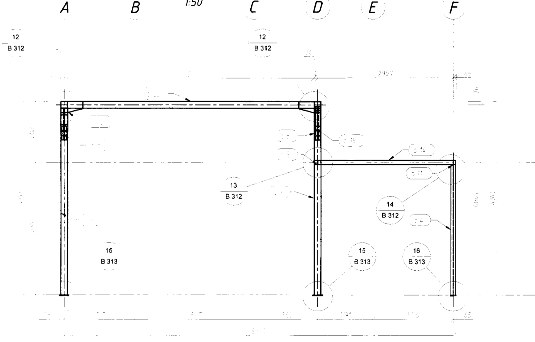
Mátlína 8 Ásýnd 1:50
