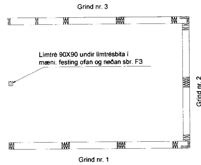
Grunnmynd veggjagrindur mkv. 1:50
