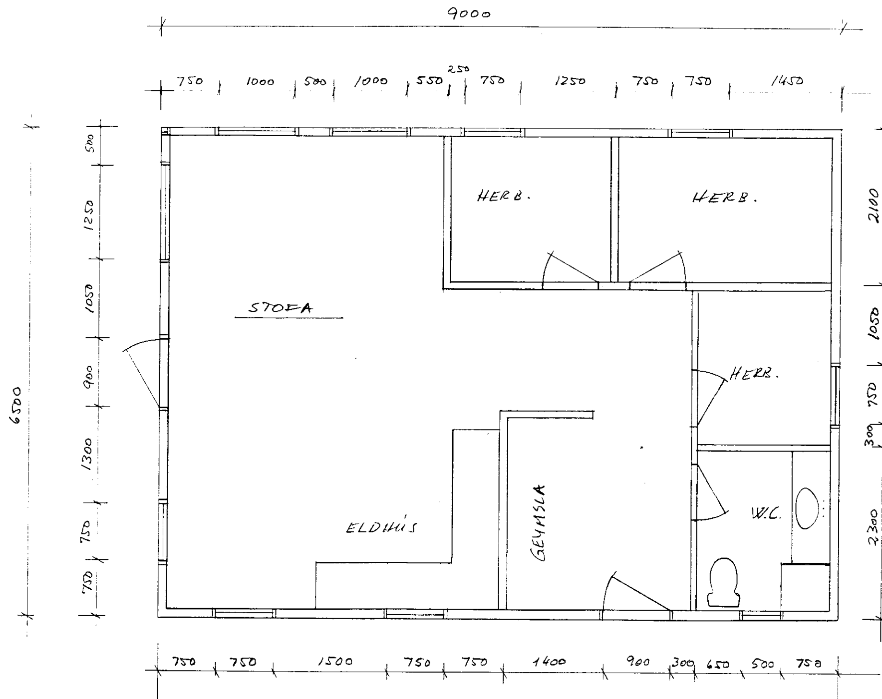
GRUNNMYND 1:50
