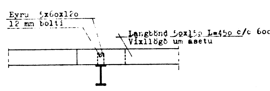
SNIF E-E 1:20 (langbönd á þaki)
