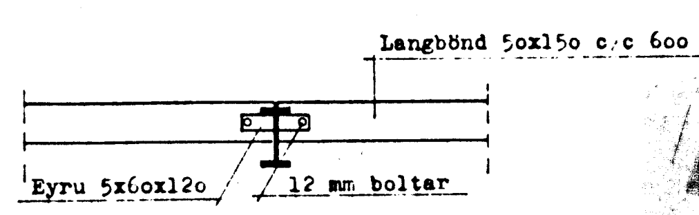
SNID F-F 1:20 (langbönd á veggjum)
