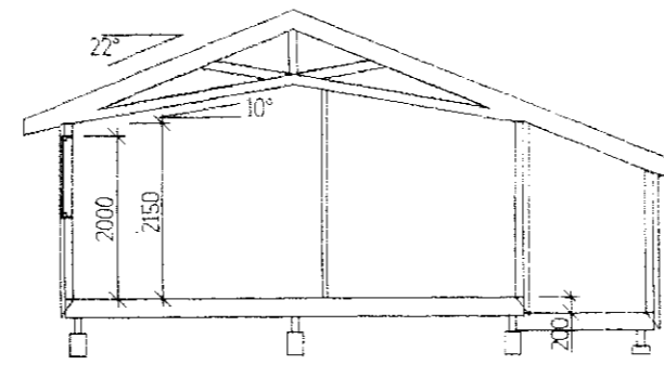
Sneidting A-A
