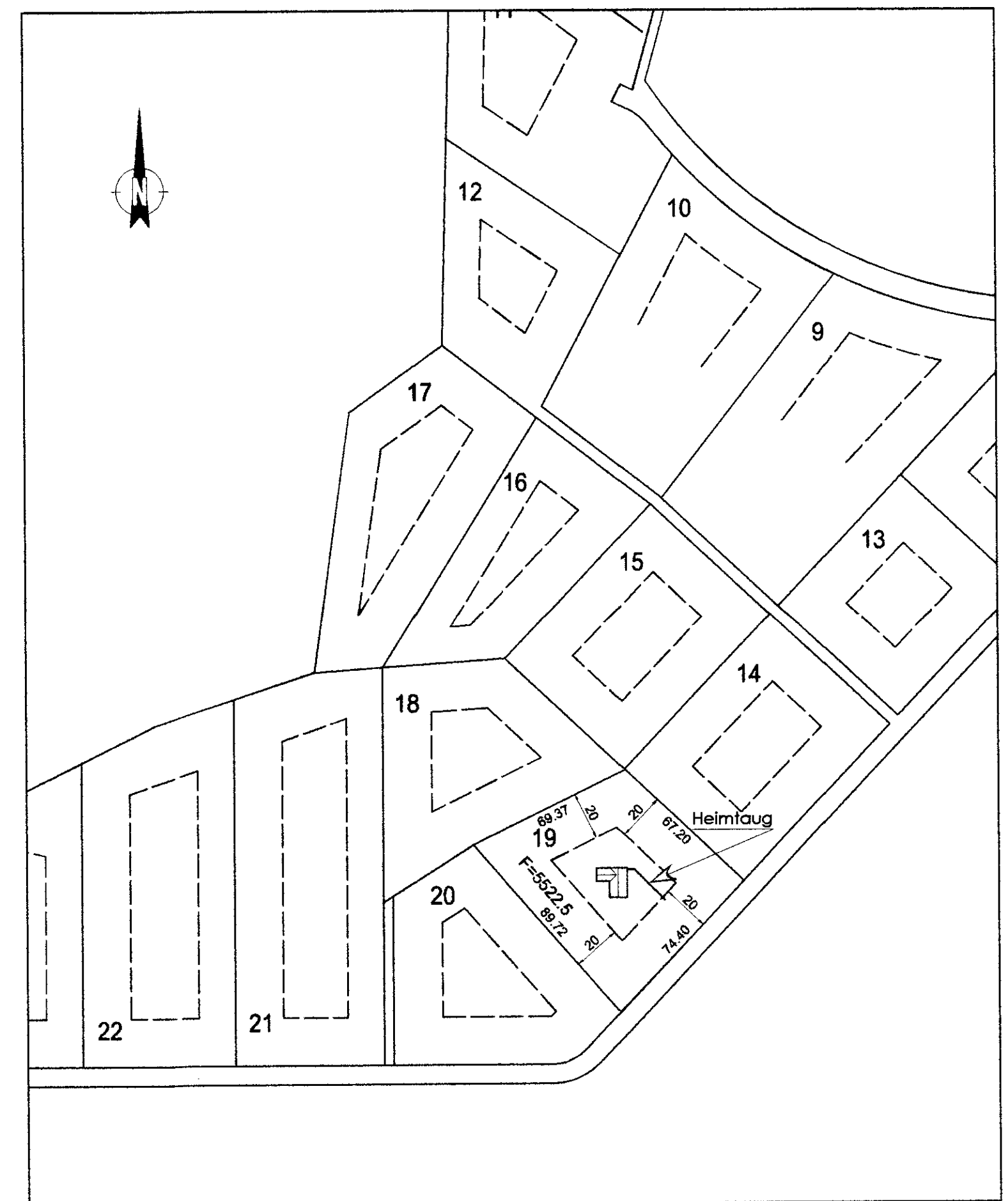
AFSTÖÐUMYND 1:1000
