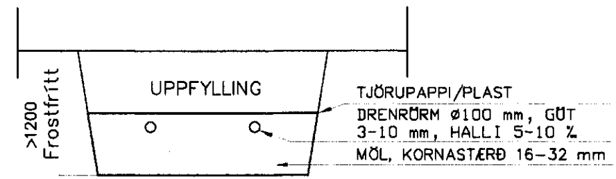
SITURLÖGN, SNIÐ A-A Mkv. 1:50
