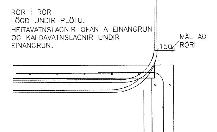
STADSETNING STÚTA VIÐ ÚTVEGG OG UNDIR PLÖTU Mkv. 1:20
