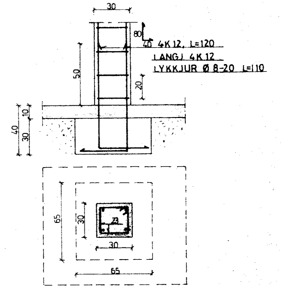
STOÐ MEÐ UNDIRST. M. 1:20
