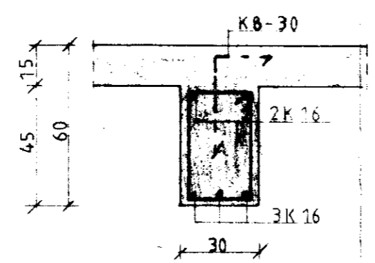
SNID A-A M=1:20
