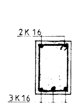
C-C M=1:20
